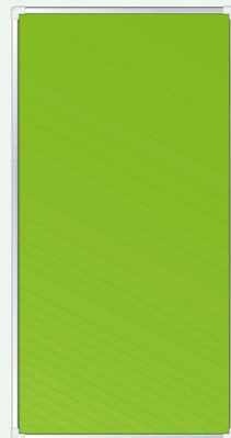
303-20 ☆ サイズ：1250×650×25mm厚 材質：耐水ベニヤ(木枠付アルミ縁) 〈付属品〉 L字型取付金具4個
